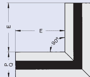
90° mitre
